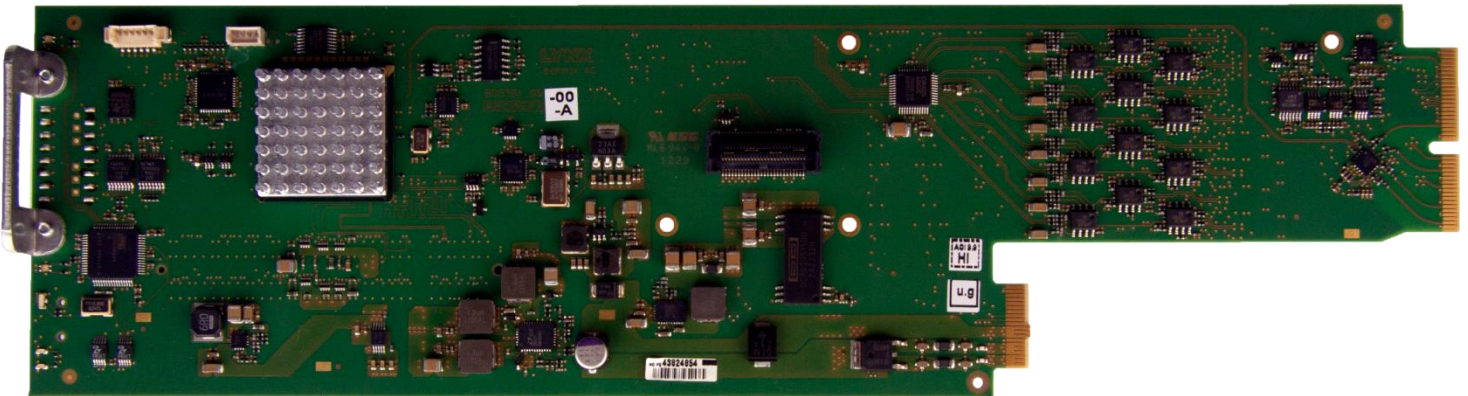
CardModule Layout
